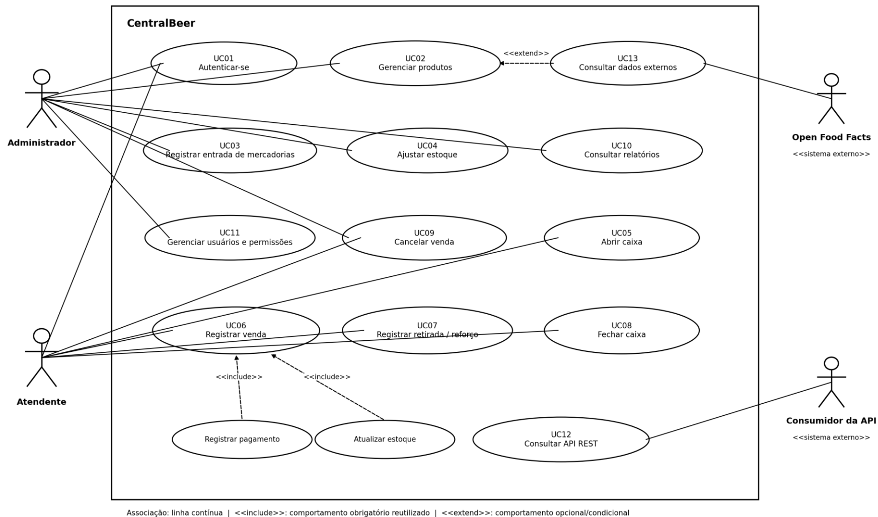
Figura 1 - Diagrama geral de casos de uso do CentralBeer. Fonte: elaboração própria com base na documentação do projeto (2026).
